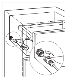
Cavo di controllo (cassetti).
