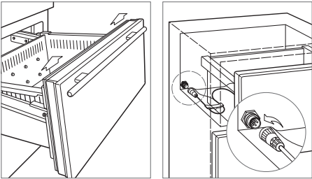
Extracción de los cajones. Cable de control (cajones).
