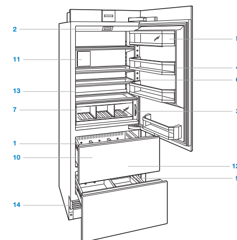
Hohe Kombination
