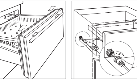
抽屉拆卸。 控制电缆（抽屉）。
