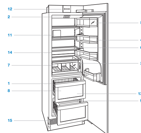
Säulenkombinationsmodell
