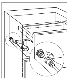
Steuerkabel (Modell ICB427RG)
