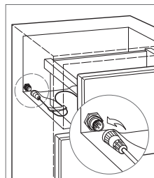
Câble de commande (Modèle ICB427RG).
